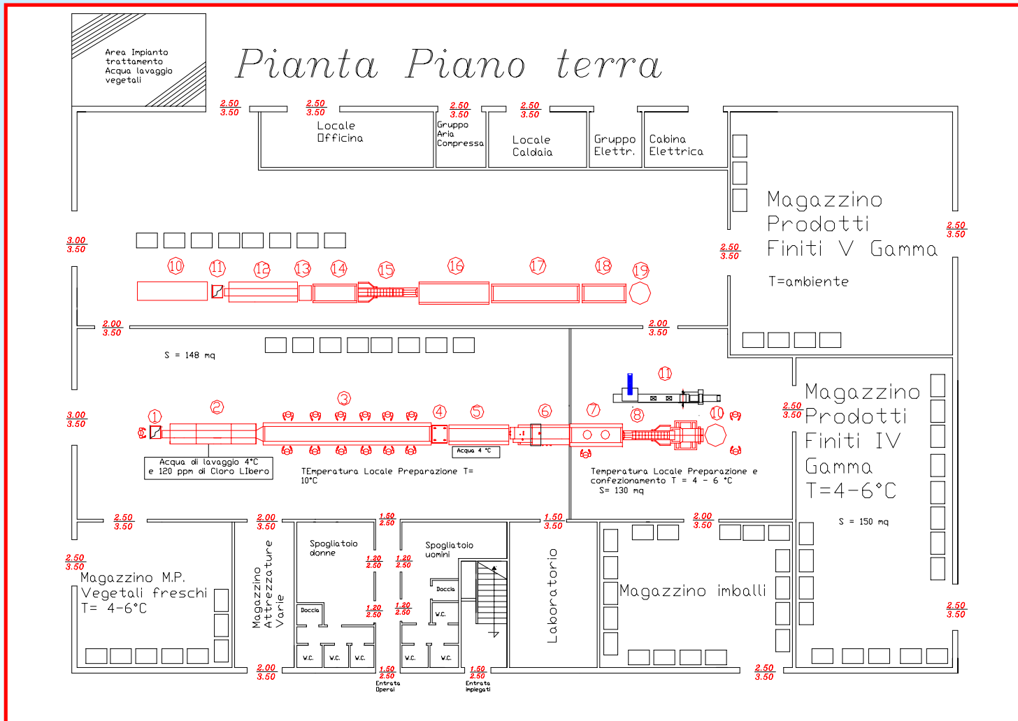
Studio e progettazione del lay-out di un impianto per la produzione di prodotti di IV e V Gamma (Società Verdivoglie (RC))
