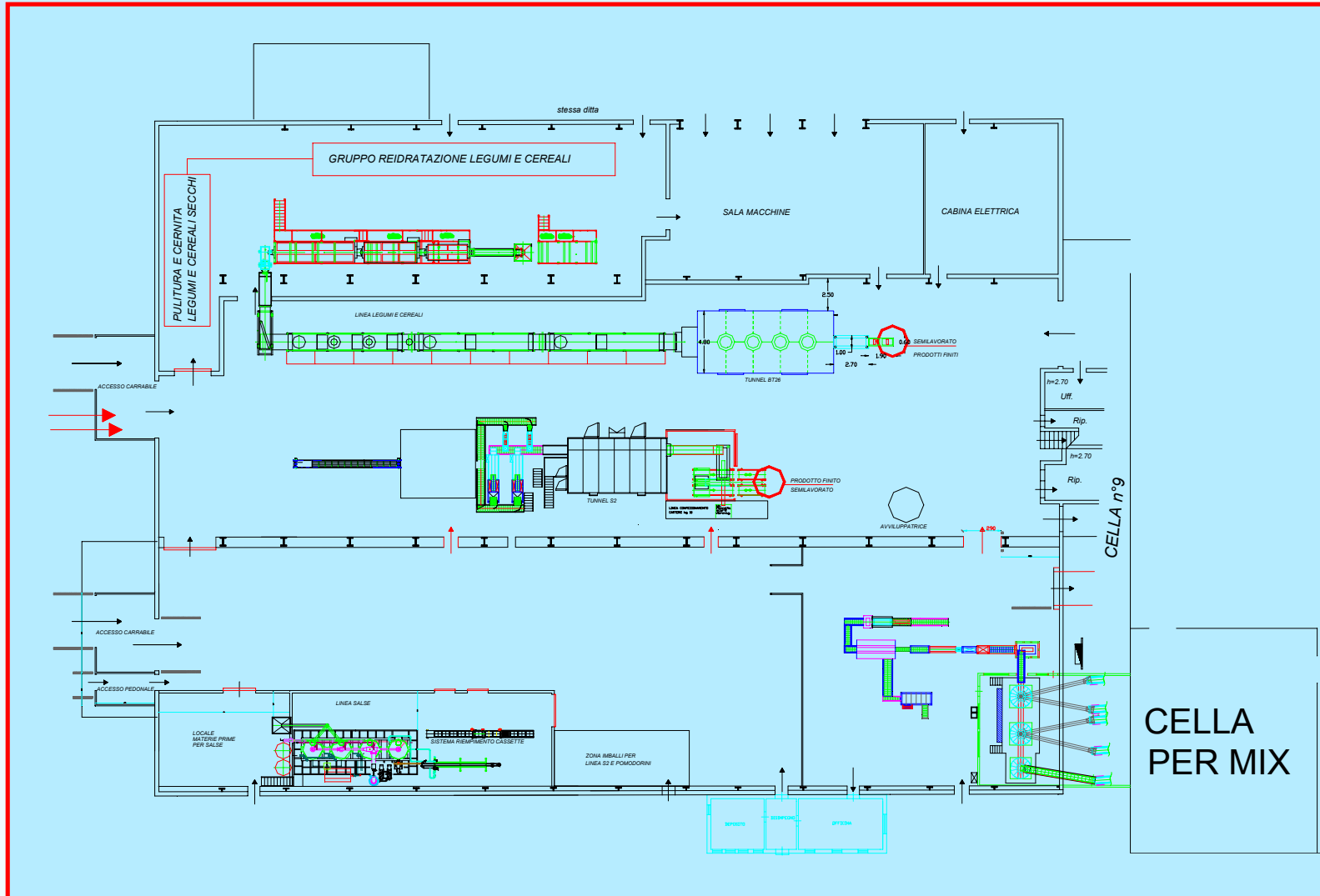
Studio e progettazione del lay-out di un impianto per la produzione di prodotti vegetali surgelati (Gruppo GIAS S.p.A. – Mongrassano Scalo (CS))
