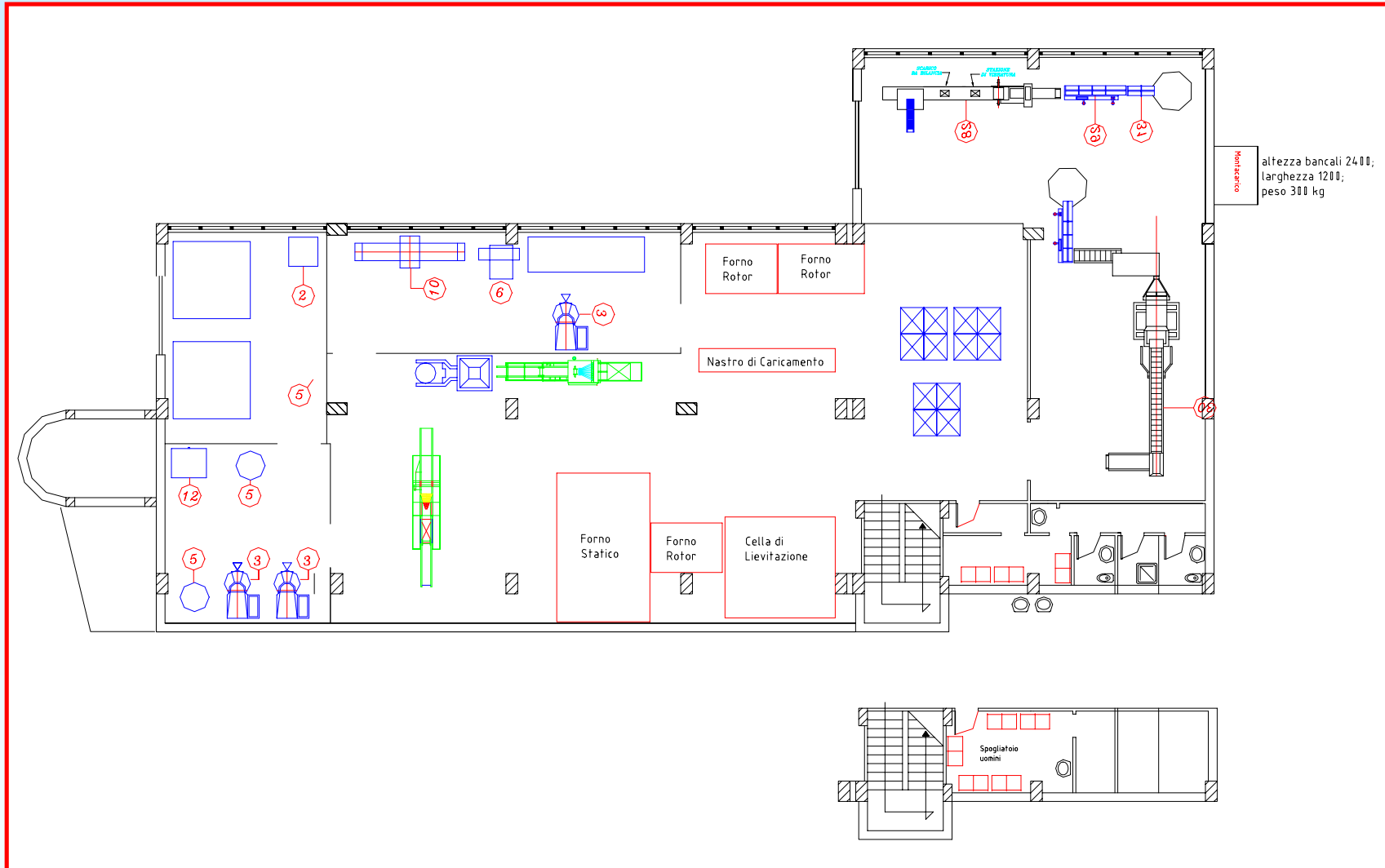
Studio e progettazione del lay-out di un impianto per la produzione di sostituti del pane e prodotti di pasticceria secca (Panificio PASCUZZO S.n.C. Parenti (CS))
